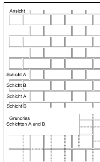
Gotischer Verband
