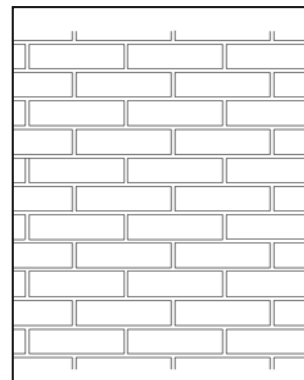
Läuferverband Steinhöhe 6,5 cm
