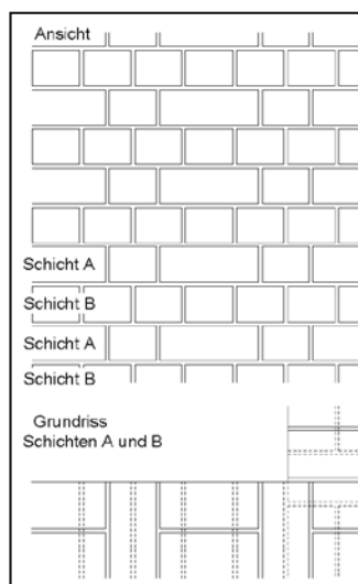
Holländerverband
