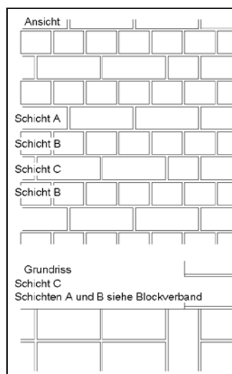
Kreuzverband
