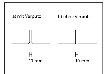
Offenes Fugensystem
